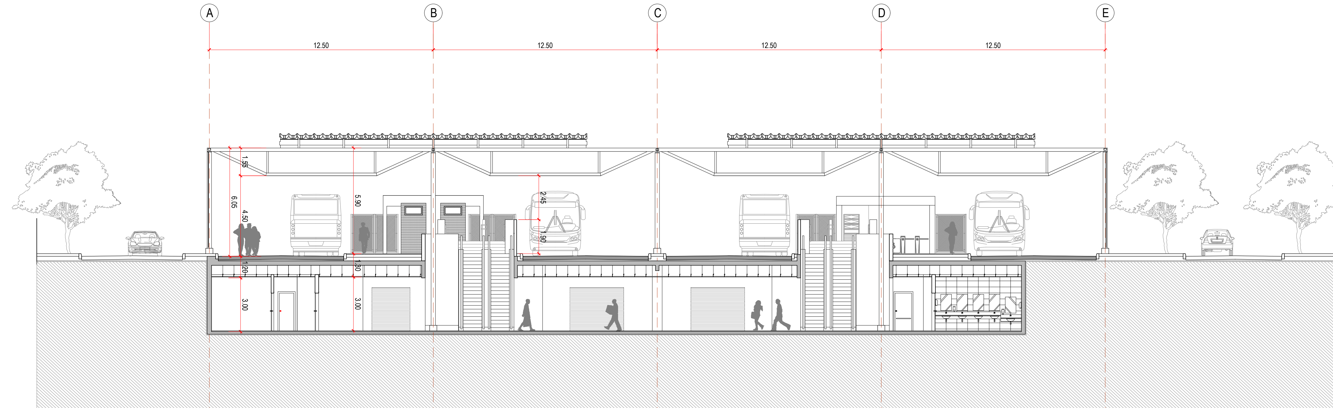
CORTE AA
